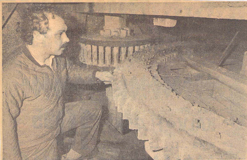
Møllebygger Jens Jørgensen på øverste gulv ved en central del af møllens maskineri, det store tandhjul, der er knapt tre meter i diameter og har 120 tænder. (Foto: Tage Jensen)
