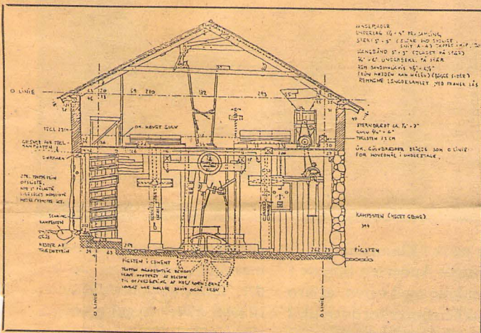
Tværsnit af vandmøllen i Bangsbostrand efter opmåling af arkitekt Roald Nordkap.
