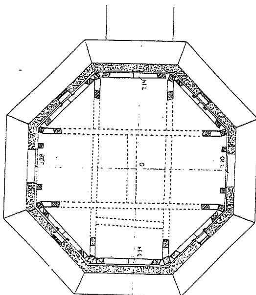
plan snit D - hatloft - mål 1:100
