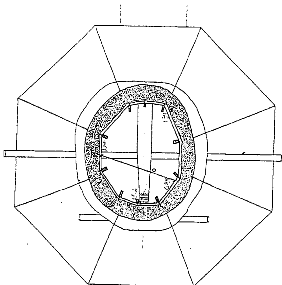
plan snit D - hatloft - mål 1:100
